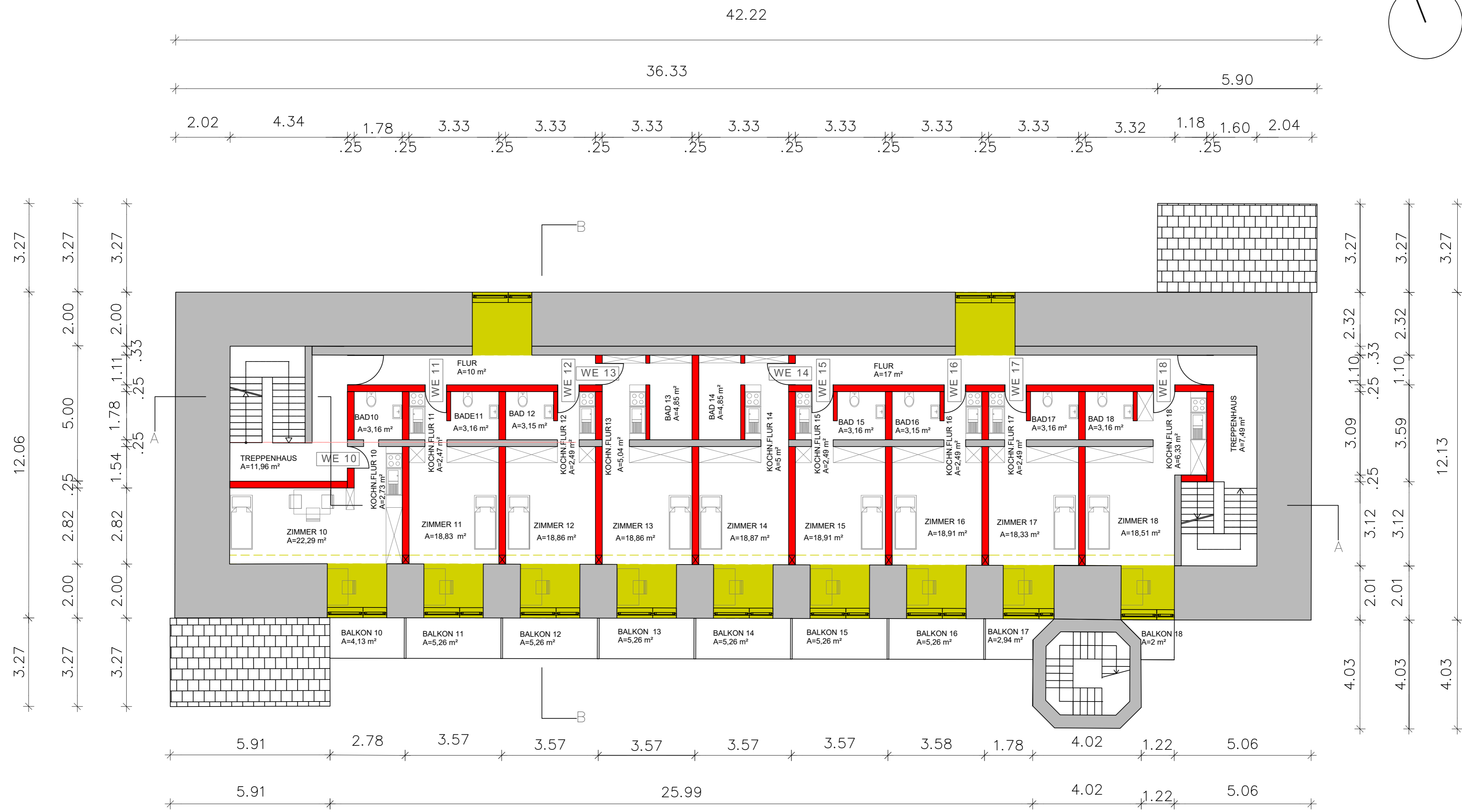
GRUNDRISS OBERGESCHOSS M 1:100 11.07.2018
